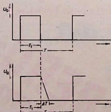
Bild 9. Die Schaltflanken beeinflussen den Mittelwert der Ausgangsspannung
