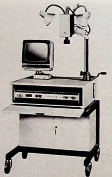
AV-Wagen „Video“ von Grundig mit einer Kamera auf höherverstellbarem, schwenk- und neigbarem Kugelstall, einem drehbaren Monitor, Bedlengerät und Beleuchtungseinrichtung
