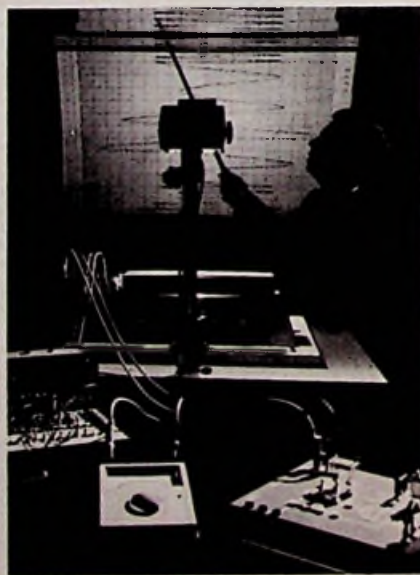
Selbstabgleichender Linienschreiber mit Overhead-Projektionseinrichtung von Siemens
