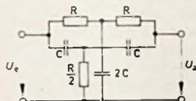
Bild 7. Schaltung zur Berechnung der Doppel-T-Filter
