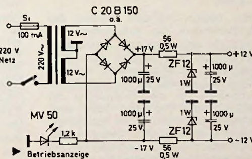
Bild 8. Stromlaufplan des stabilisierten Netzteils
