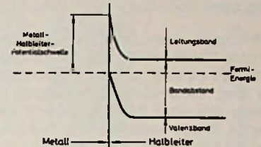
Bild 1. Bändermodell eines Metall-Halbleiter-Überganges. Die Elektronen im Metall haben Energien unter der Fermi-Energie
