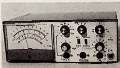
Bild 1. Ansicht des NF-Millivoltmeters mit Klirrfaktor-Meßzusatz
