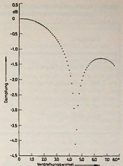
Bild 2. Spannungs- und Phasendämpfung als Funktion des Spalt-Verdrehungswinkels (Computer-Ausdruck; die Skalenwerte der x-Achse sind mit 0,1, die der y-Achse mit 10 zu multiplizieren)
