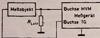
Bild 10. Prinzip der Klirrfaktormessung
